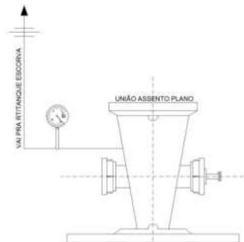
Figura C.6 – Arrefecimento da bomba principal elétrica
