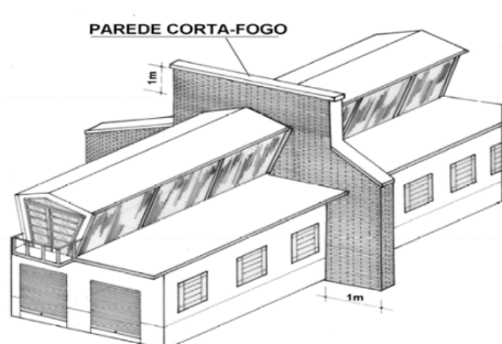
Figura 8 – Parede corta-fogo
