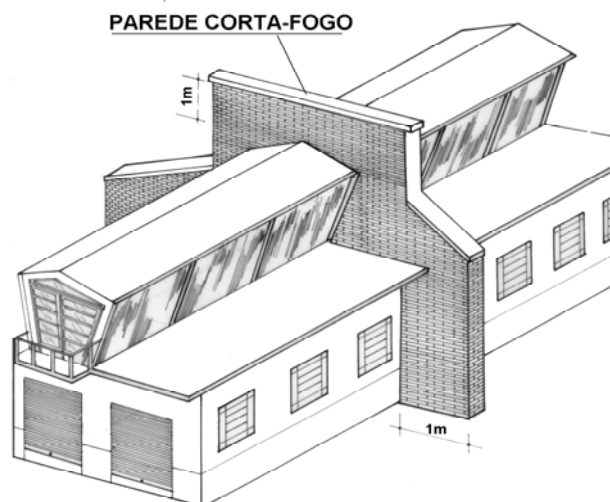
Figura 8 - Parede corta fogo
