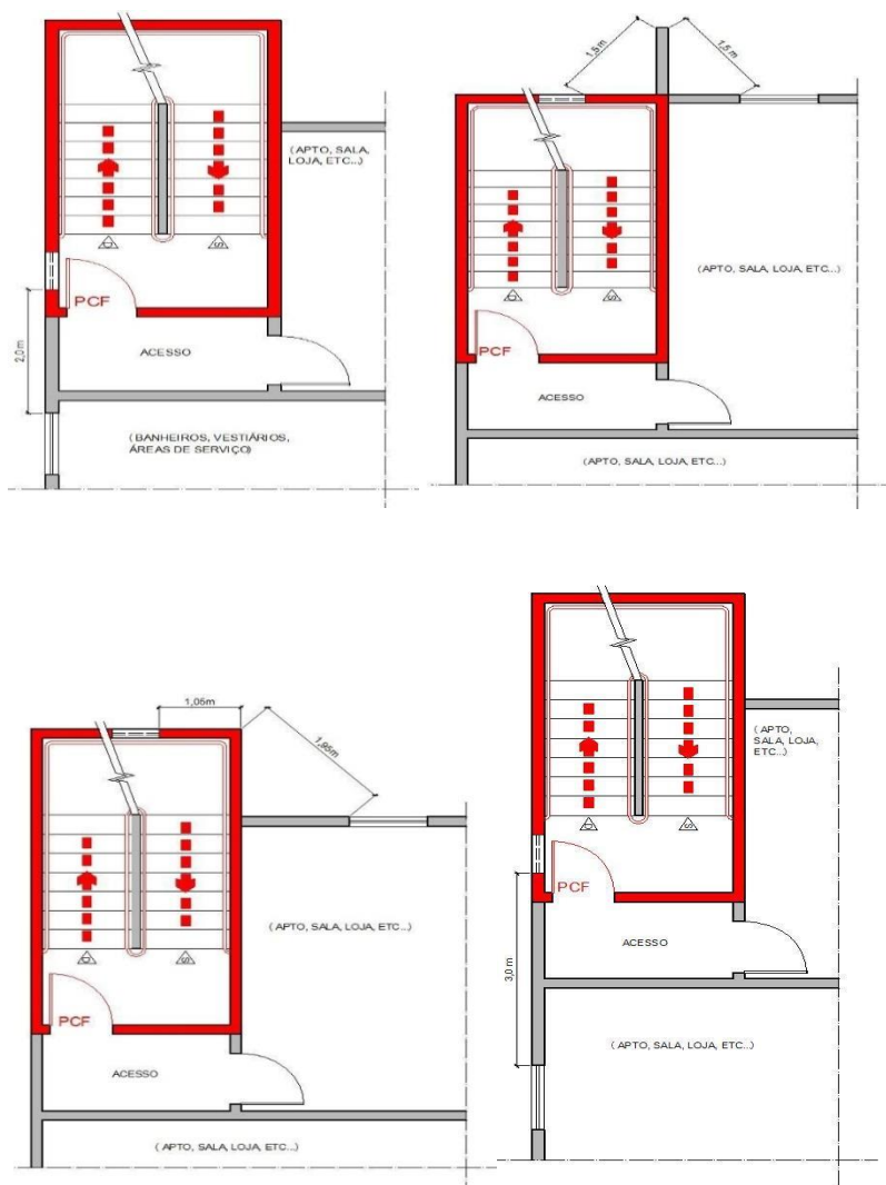
Figura 11 – Exemplos de distância entre janelas de escadas protegidas e outras aberturas
