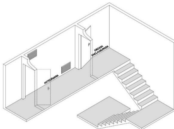
Figura 14 – Antecâmaras e Duto de ar – Desenho esquemático
