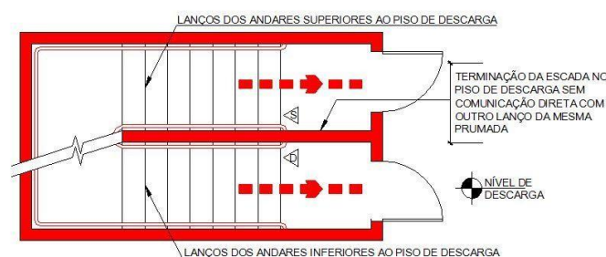
Figura 3 – Segmentação das escadas no piso da descarga
