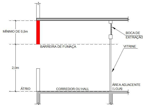
Figura 4: Detalhe de barreira de fumaça – corte
