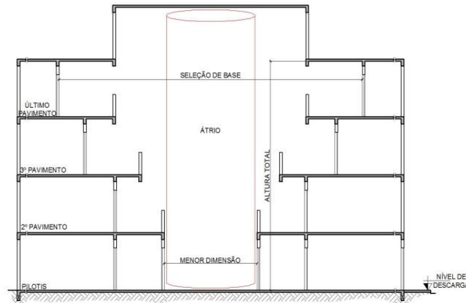
Figura 28 – Exemplo de átrio não padronizado
