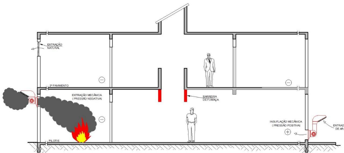
Figura 12 – Exemplo de controle de fumaça por controle mecânico e entrada de ar mecânica
