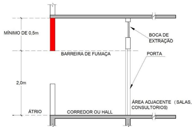
Figura 30 – Exemplo de locais fechados com acesso à circulação por meio de uma porta
