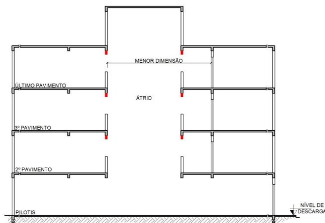
Figura 23 – Átrio coberto aberto
