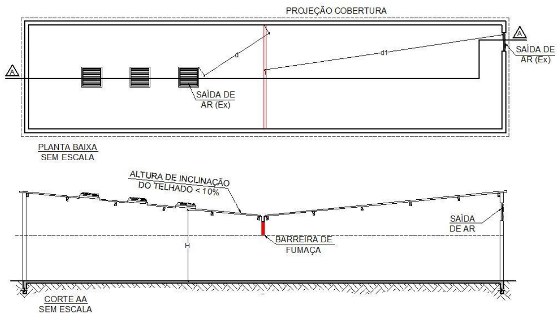
Figura 5 – Distâncias entre saídas
