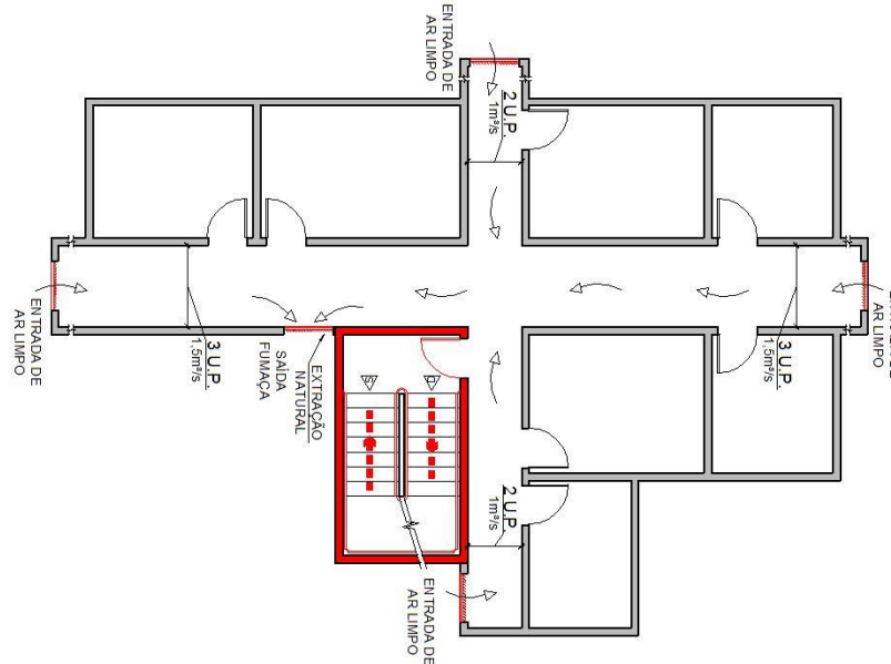
Figura 20 – Rotas de fuga com largura variável
