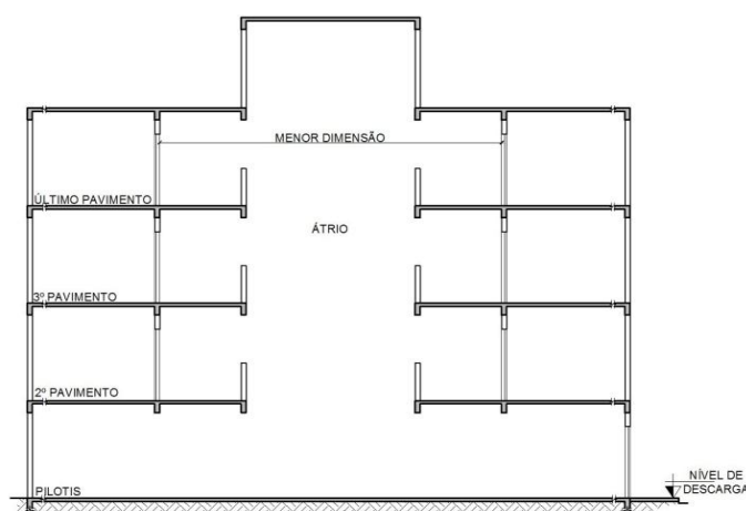
Figura 25 – Modelo 2 de átrios cobertos fechados
