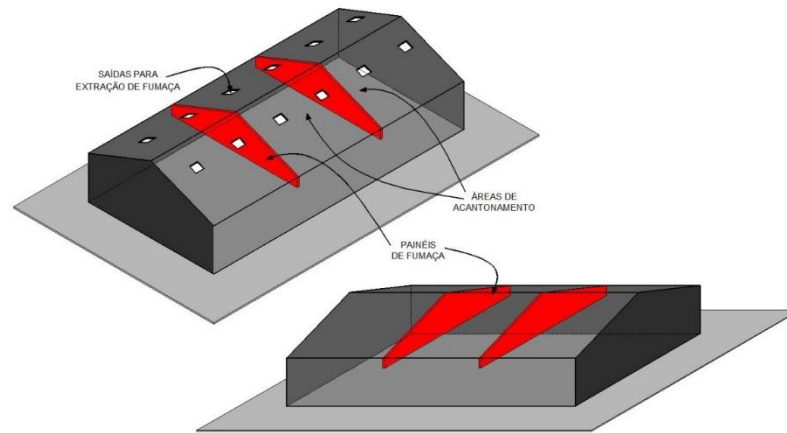
Figura 2 – Elementos do sistema de controle de fumaça
