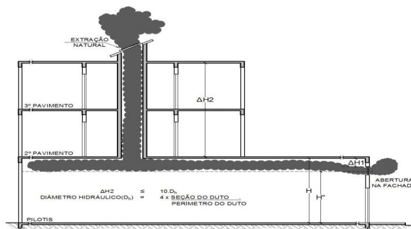
Figura 8 – Diâmetro hidráulico
