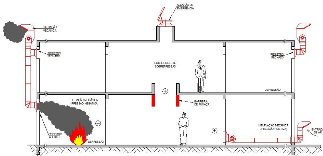
Figura 21 – Controle por sobrepressão
