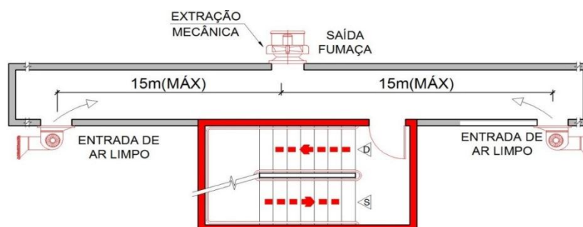
Figura 18 a – Distância em linha reta de aberturas de extração para Tipo 2
