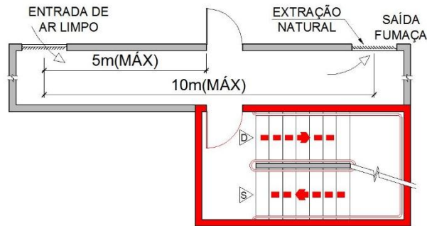
Figura 17 – Distância de entrada de ar de portas de acesso
