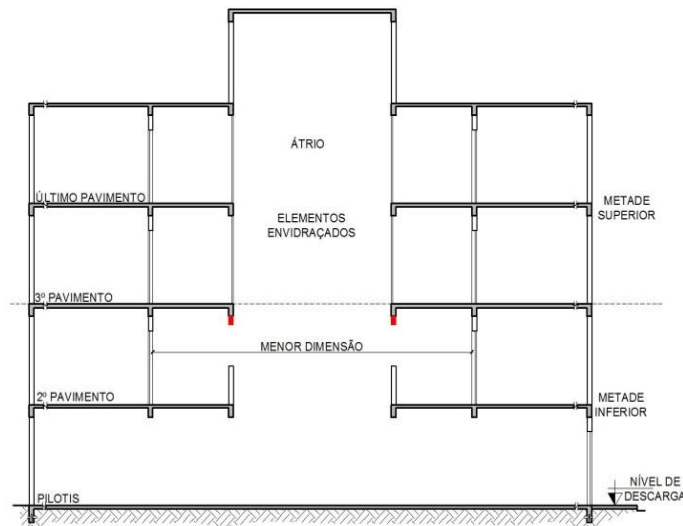
Figura 29 – Fechamento do átrio
