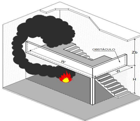
Figura 13 – Dados e parâmetros utilizados para equação 8
