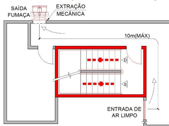
Figura 19 b – Distância de extração de aberturas em trajeto diverso tipo 3
