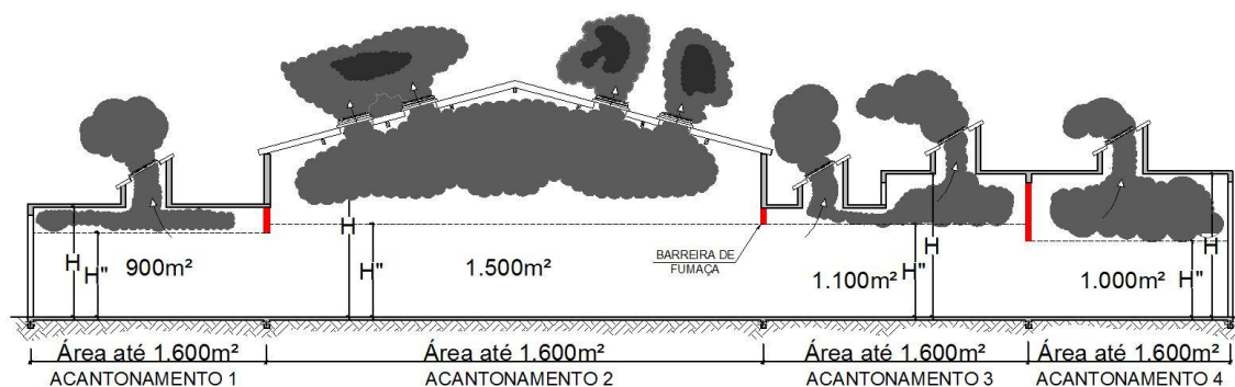
Figura 6 – Altura de referência diversificada por acantonamento
