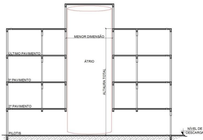
Figura 27 – Dados relativos a um átrio coberto padronizado
