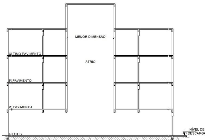
Figura 24 – Modelo 1 de átrios cobertos fechados
