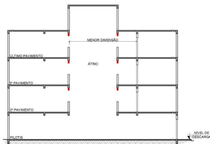
Figura 26 – Átrio considerado aberto de um lado e fechado do outro
