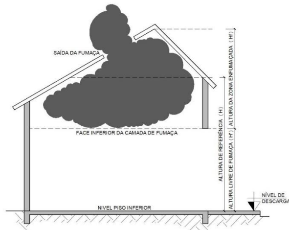
Figura 3 – Altura de referência, altura livre de fumaça e zona enfumaçada
