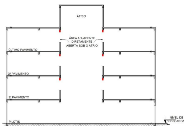
Figura 32 – Exemplo de locais diretamente abertos sob o átrio
