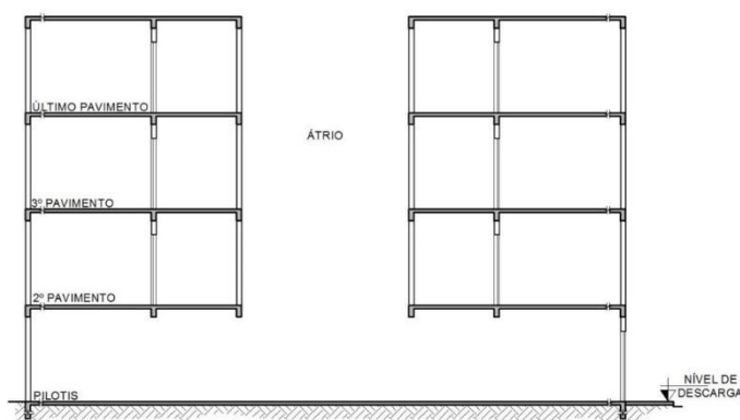
Figura 22 – Átrio ao ar livre
