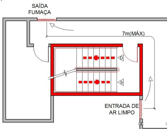
Figura 16 – Distância de extração de aberturas em trajeto diverso
