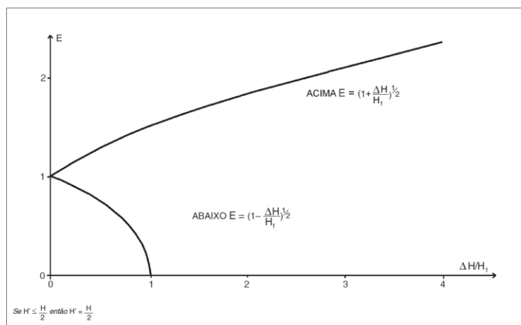
Figura 7 – Eficiência dos Exaustores
