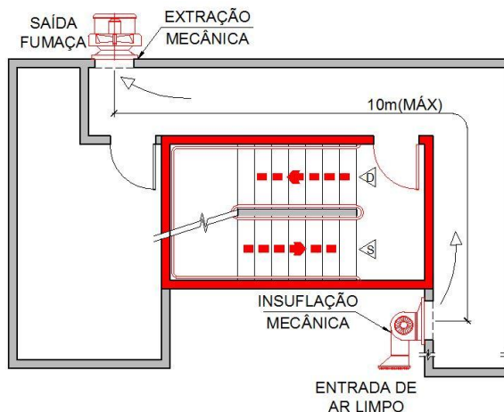
Figura 19 a – Distância de extração de aberturas em trajeto diverso tipo 2.
