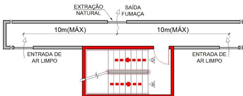
Figura 15 – Distância em linha reta de aberturas de extração
