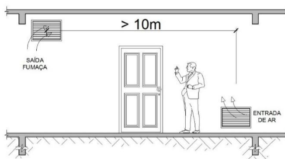
Figura 14 – Posição de aberturas de extração e entrada de ar
