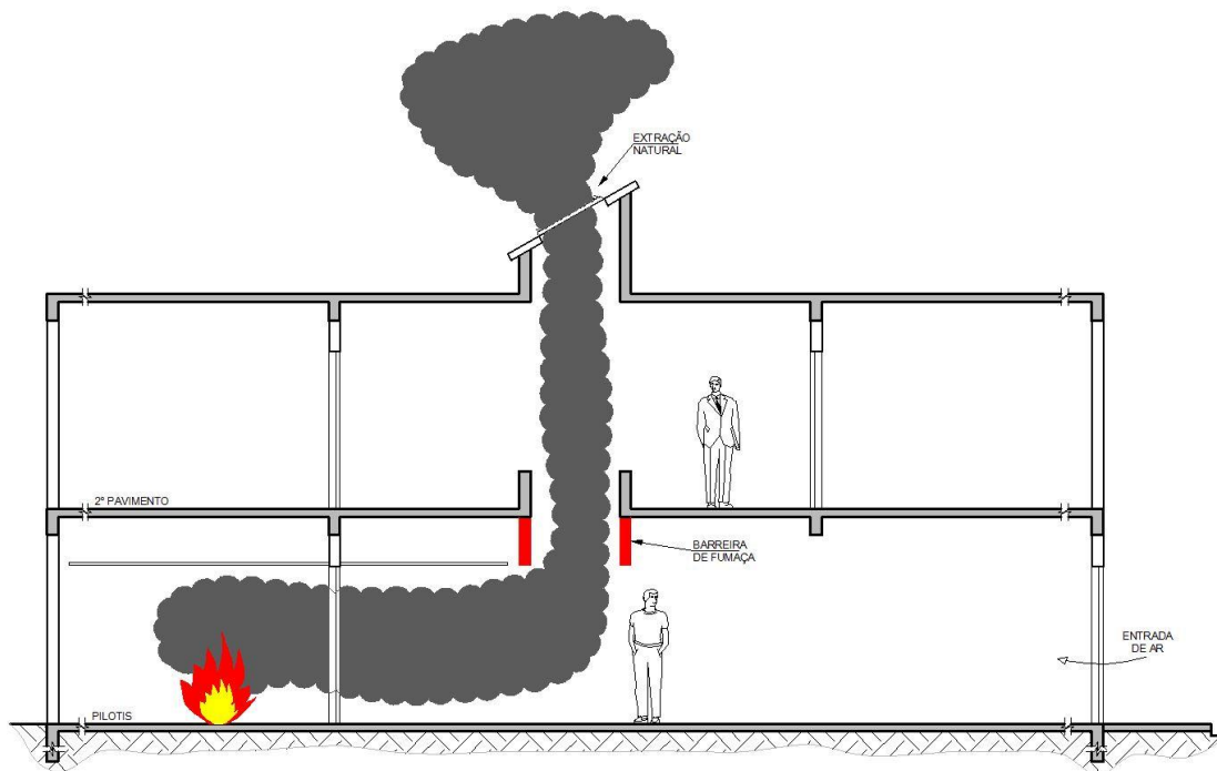
Figura 11 – Exemplo de controle de fumaça natural
