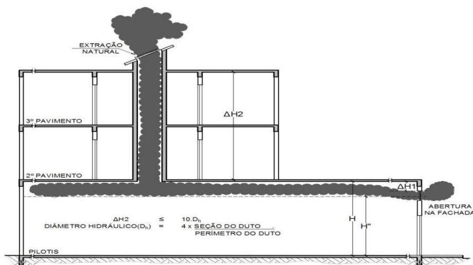
Figura 8: Diâmetro hidráulico
