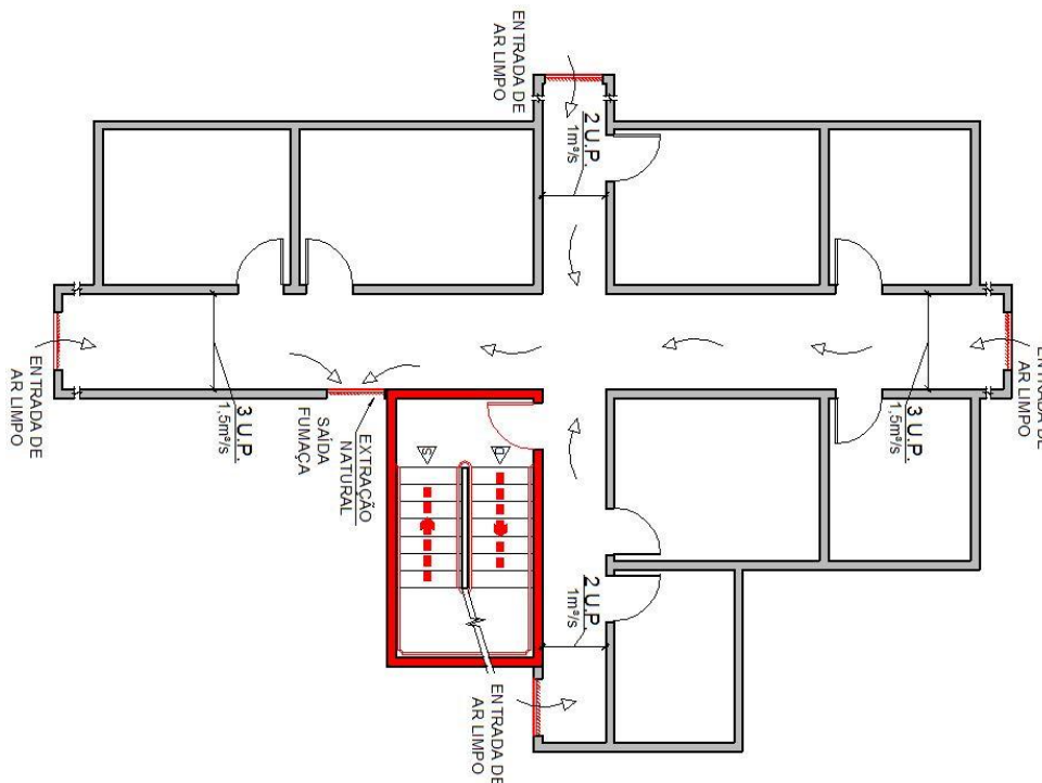
Figura 20: Rotas de fuga com largura variável
