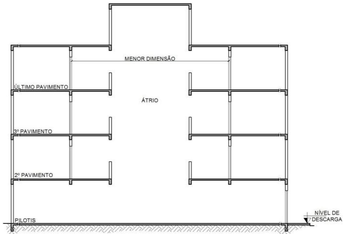
Figura 25: Modelo 2 de átrios cobertos fechados
