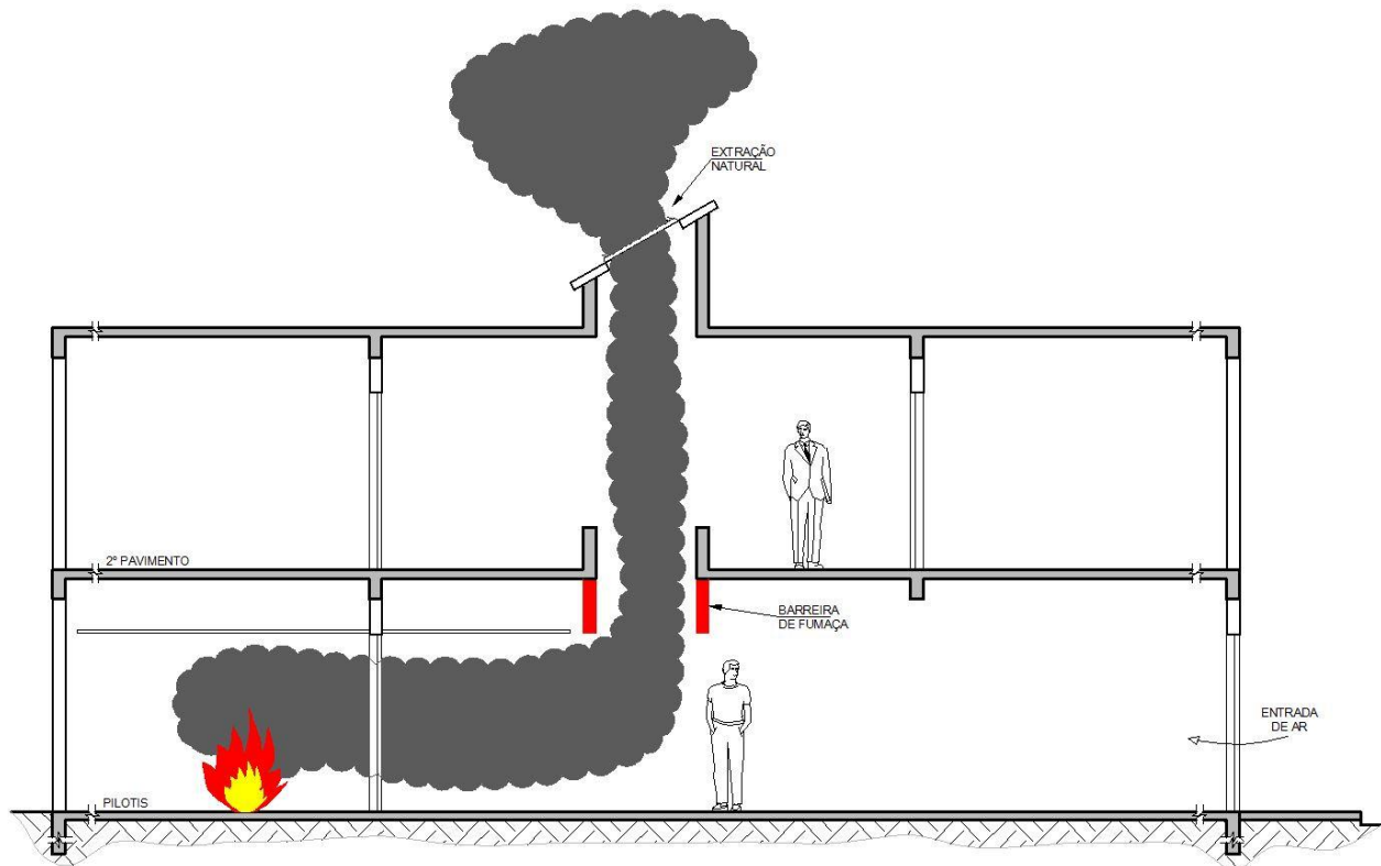
Figura 11: Exemplo de controle de fumaça natural
