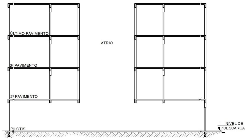
Figura 22: Átrio ao ar livre
