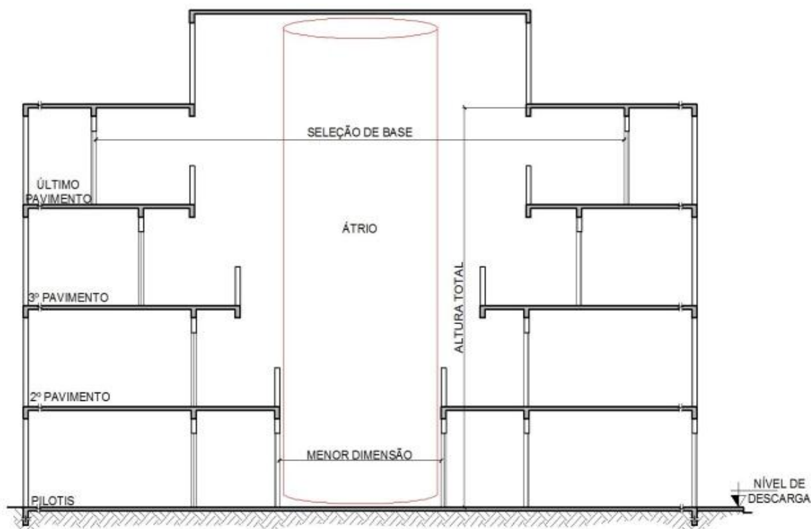
Figura 28: Exemplo de átrio não padronizado
