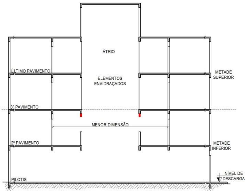
Figura 29: Fechamento do átrio
