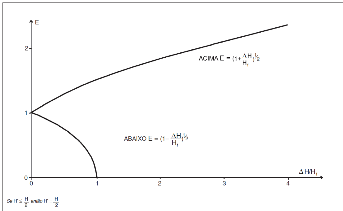
Figura 7 - Eficiência dos Exaustores
