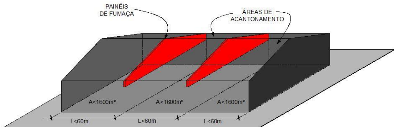
Figura 1: Divisão em áreas de acantonamento
