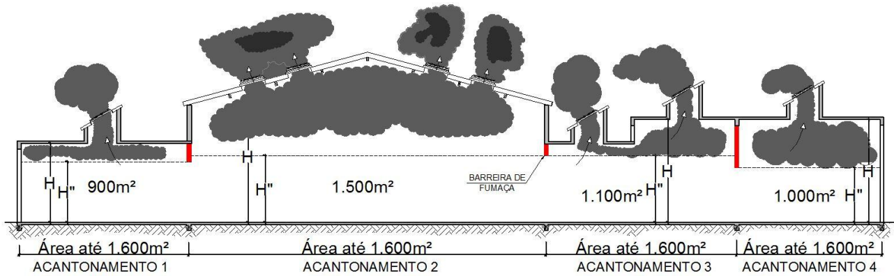
Figura 6: Altura de referência diversificada por acantonamento
