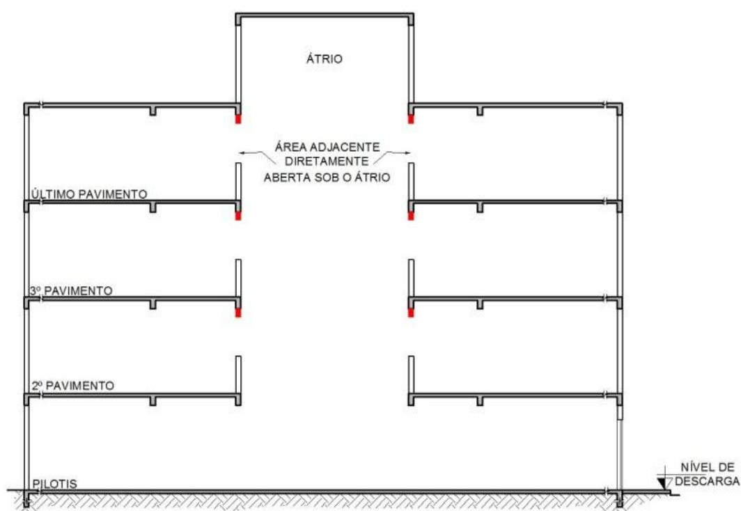
Figura 32: Exemplo de locais diretamente abertos sob o átrio
