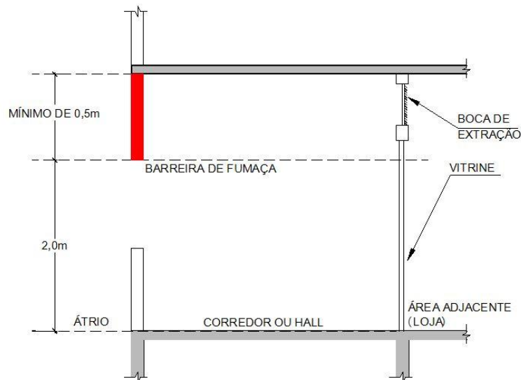
Figura 4: Detalhe de barreira de fumaça – corte
