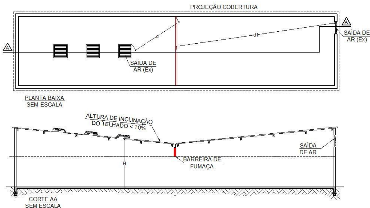
Figura 5: Distâncias entre saídas
