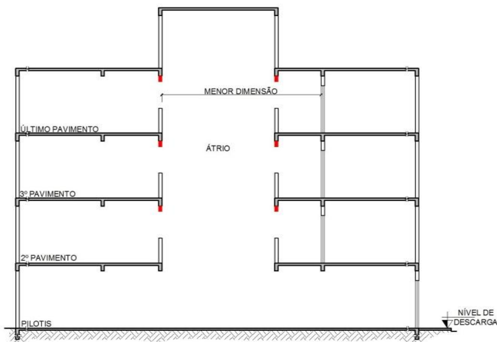
Figura 23: Átrio coberto aberto
