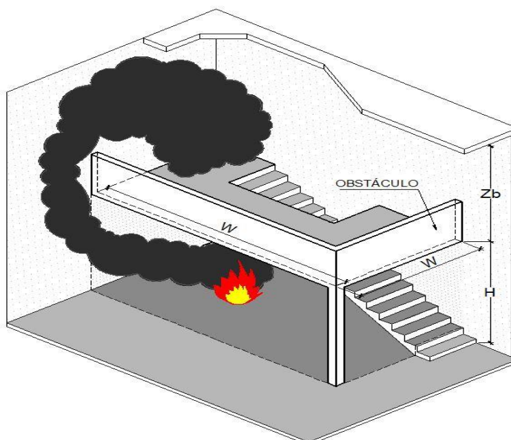
Figura 13: Dados e parâmetros utilizados para equação 8
