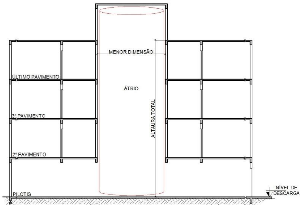
Figura 27: Dados relativos a um átrio coberto padronizado
