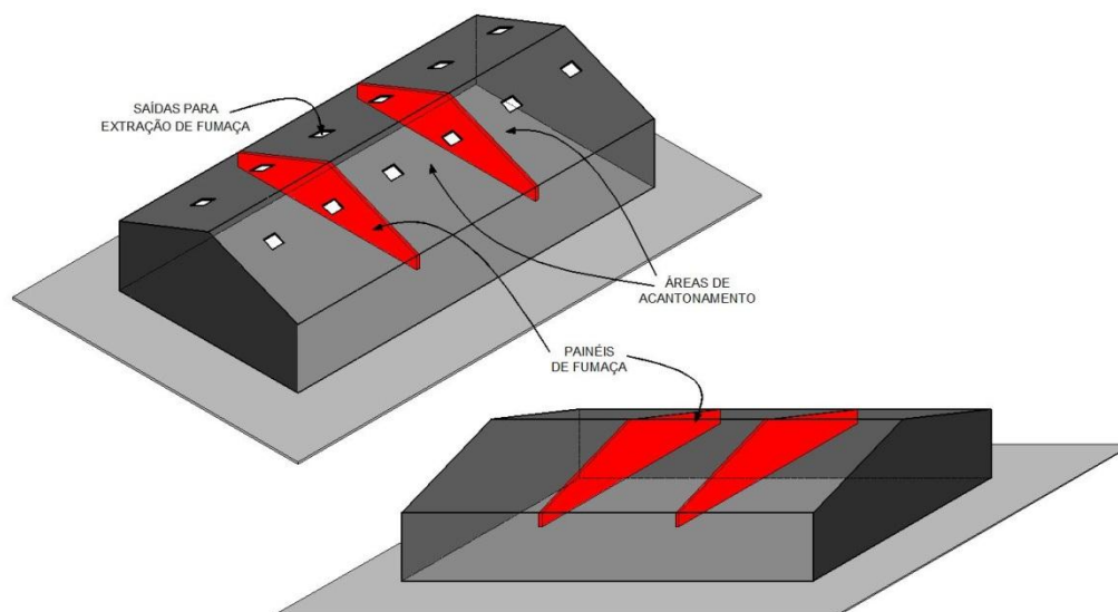
Figura 2: Elementos do sistema de controle de fumaça
