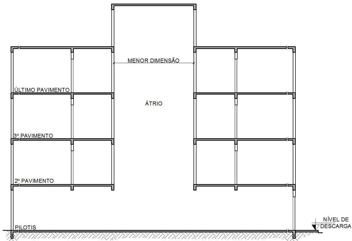
Figura 24: Modelo 1 de átrios cobertos fechados
