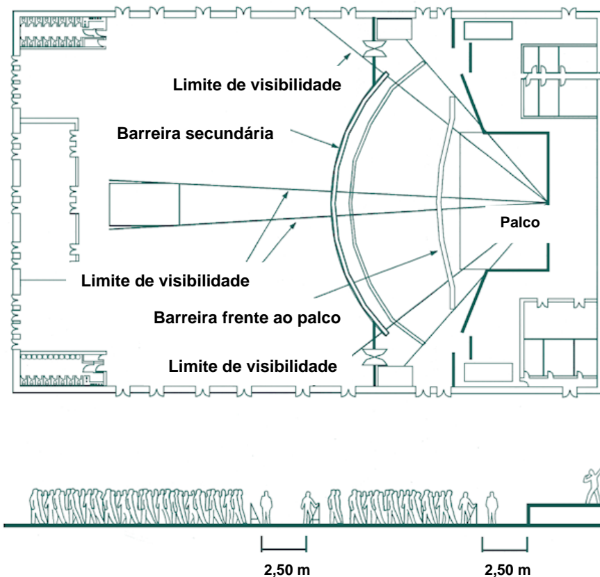
Figura nº 04: Setorização com barreiras antiesmagamento dentro de edificação
