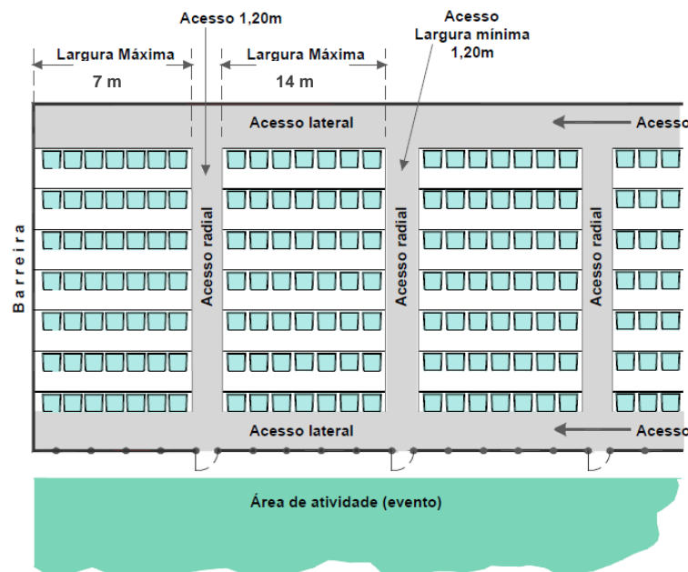
Figura nº 9: Arquibancada provisória
