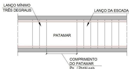
Figura 7 – Lanço mínimo e comprimento dos patamares
