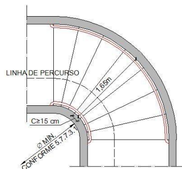
Figura 8 – Escada NE curva admissível como saída de emergência
