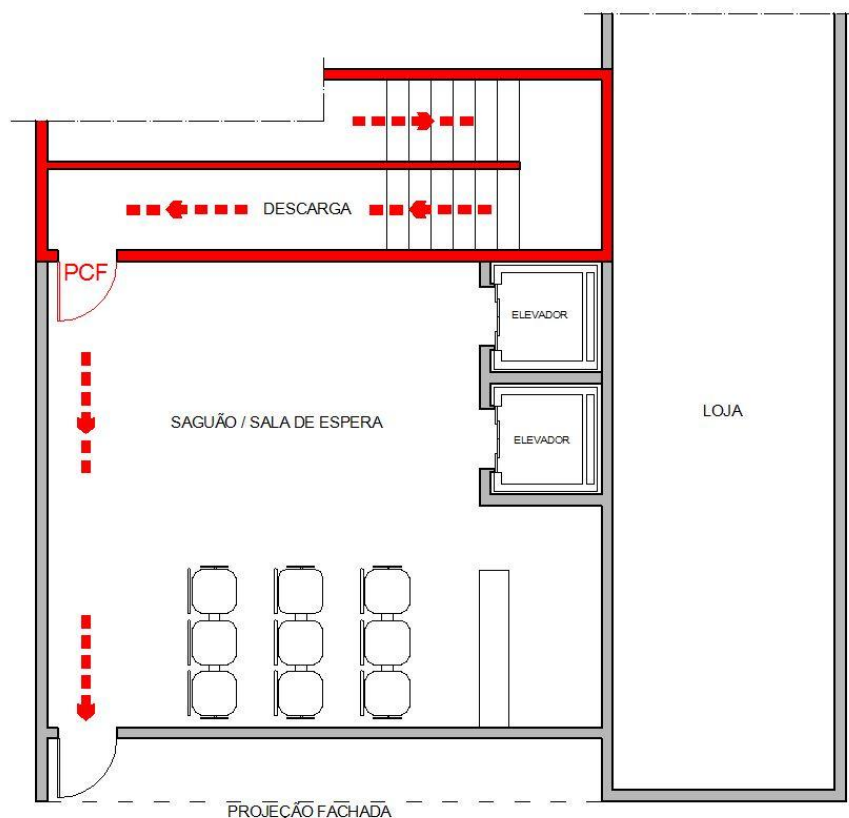
Figura 22 - Descarga através de hall térreo não enclausurado
