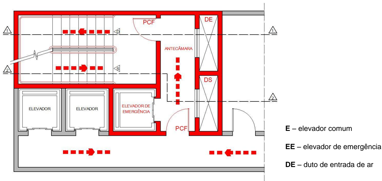
Figura 12 - Escada enclausurada à prova de fumaça, com elevador de emergência (posição exemplificativa) na antecâmara.
