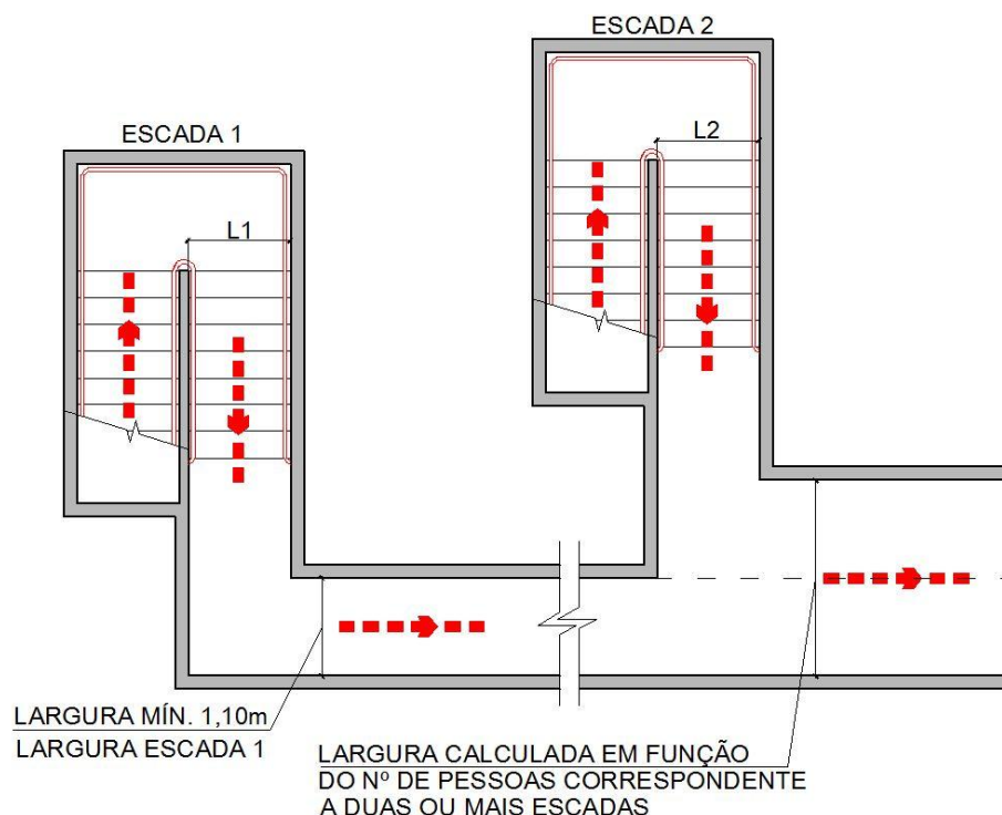
Figura 23 – Dimensionamento de corredores de descarga
