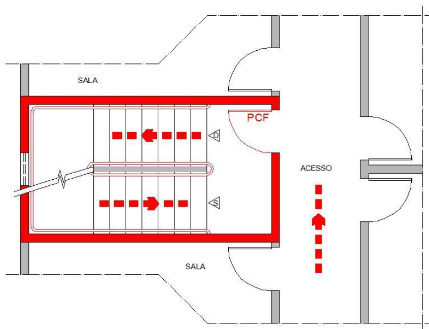
Figura 9 Escada enclausurada protegida, caso normal 5.7.8.1.
