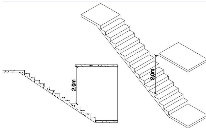
Figura 4 – Altura mínima de pé direito
