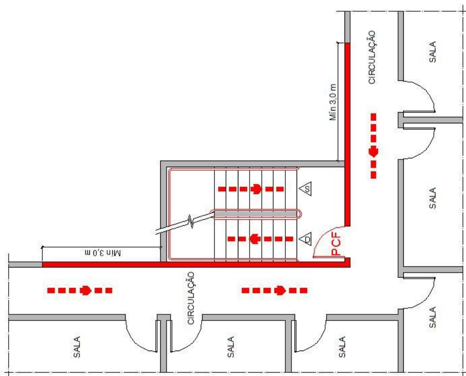
Figura 16 – Escada aberta externa
