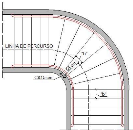
Figura 6 – Escada com lanço misto e degraus balanceados
