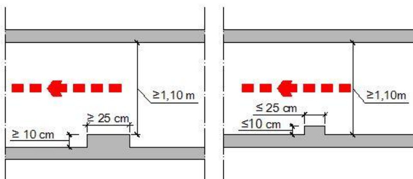
Figura 1 - Medida da largura em corredores e passagens
