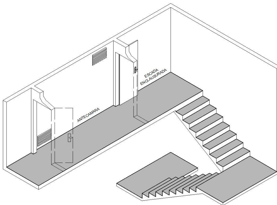
Figura 14 – Antecâmaras e Duto de ar – Desenho esquemático
