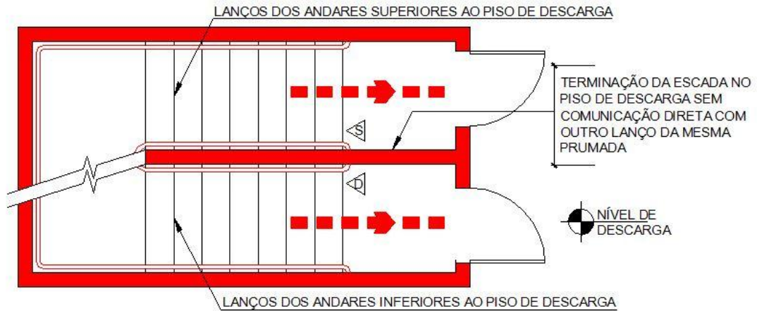
Figura 3 – Segmentação das escadas no piso da descarga
