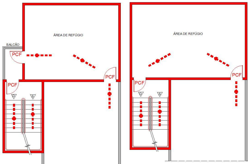
Figura 21 - Desenho esquemático da área de refúgio
