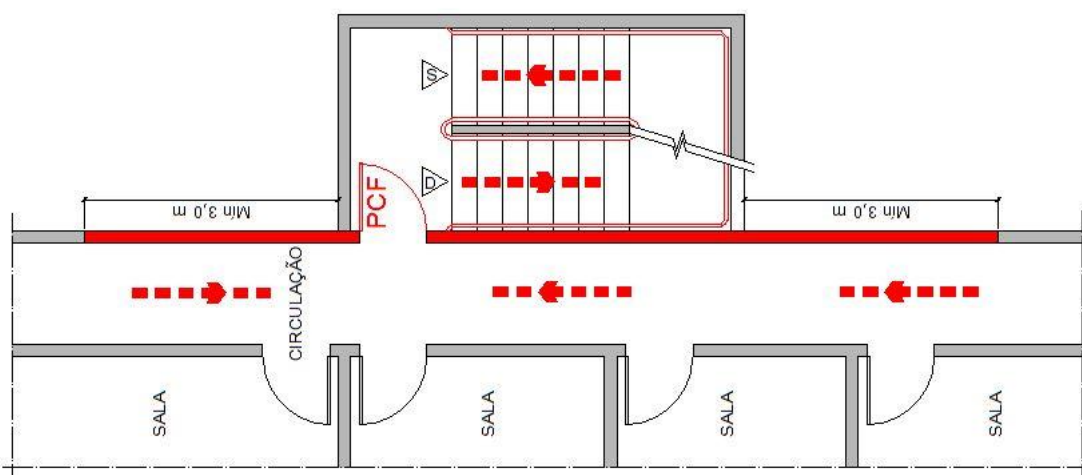
Figura 17 – Escada aberta externa
