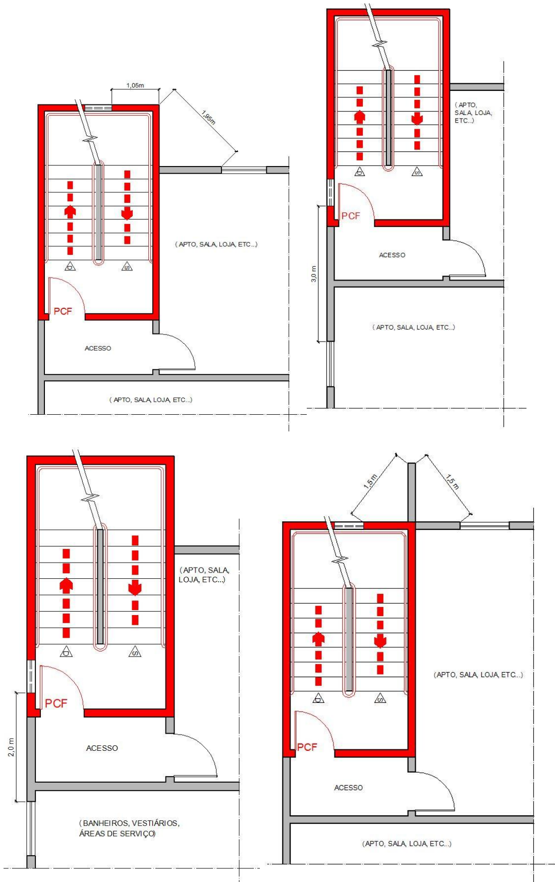
Figura 11 - Exemplos de distância entre janelas de escadas protegidas e outras aberturas
