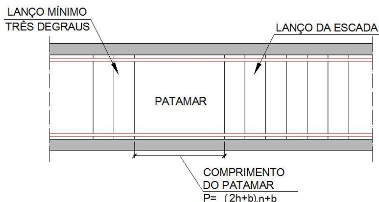
Figura 7 - Lanço mínimo e comprimento dos patamares
