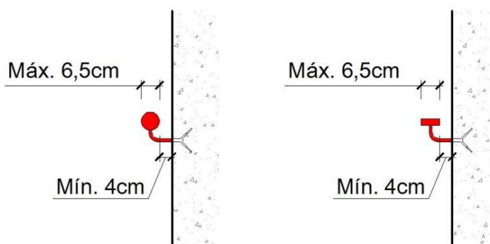
Figura 19 - Pormenores de corrimãos
