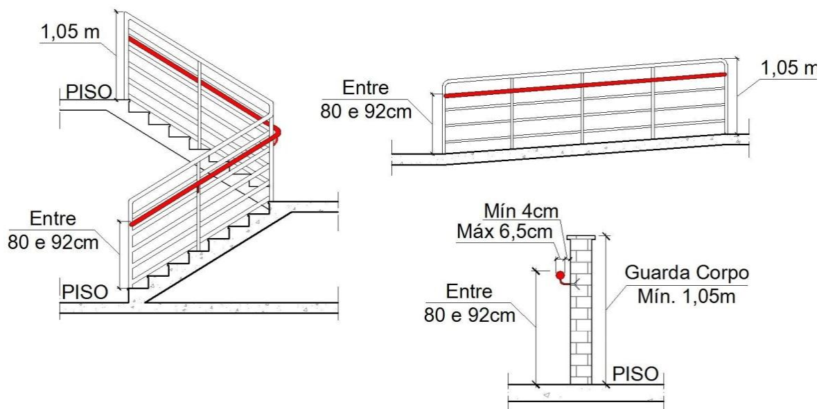
Figura 18 - Dimensões de guardas e corrimãos
