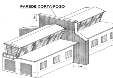
Figura 8 – Parede corta-fogo
