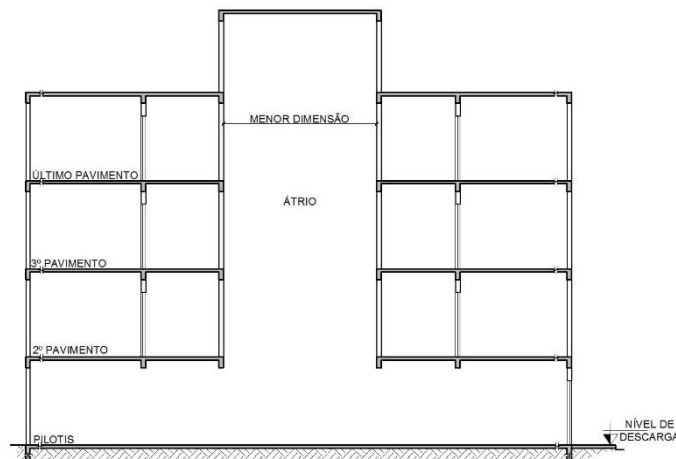
Figura 24 – Modelo 1 de átrios cobertos fechados
