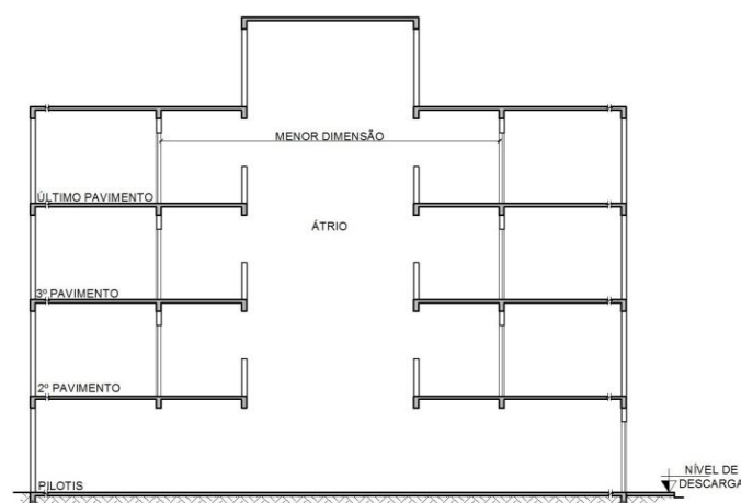
Figura 25 – Modelo 2 de átrios cobertos fechados
