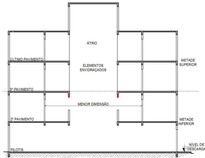
Figura 29 – Fechamento do átrio
