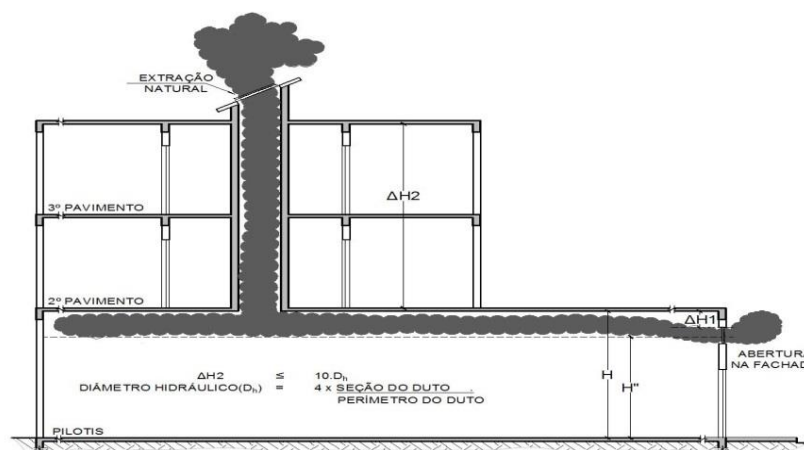
Figura 8 – Diâmetro hidráulico
