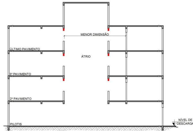
Figura 23 – Átrio coberto aberto
