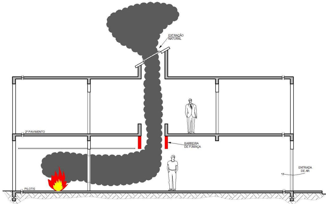
Figura 11 – Exemplo de controle de fumaça natural
