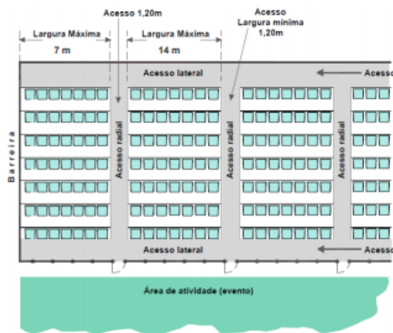
Figura H.2.2 - Arquibancada provisória
