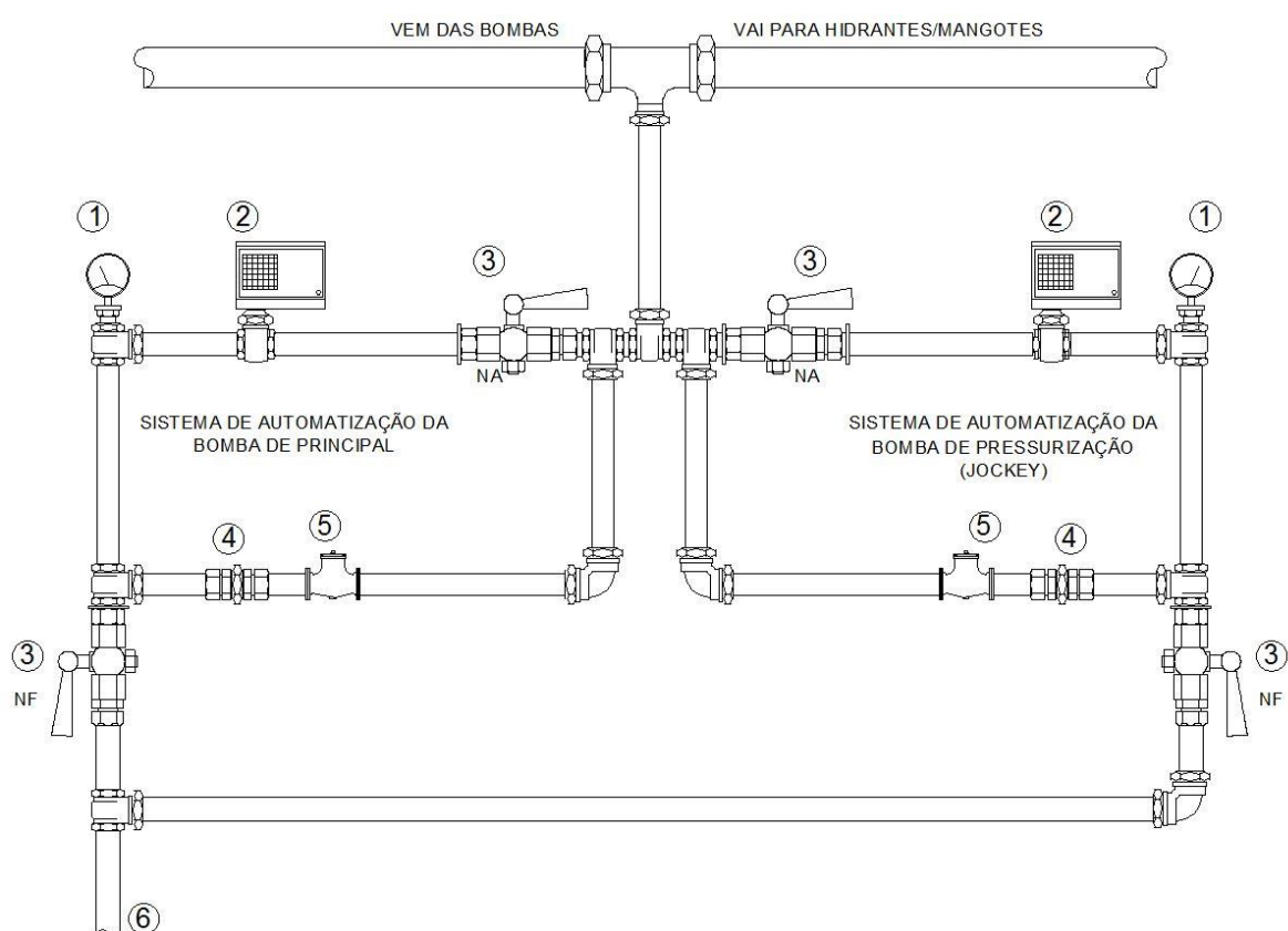
Figura C.2 – Cavalete de automação das bombas principal e de pressurização
