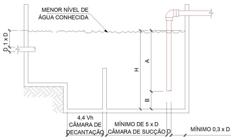
Figura B.6 - Alimentação natural de reservatório por conduto
