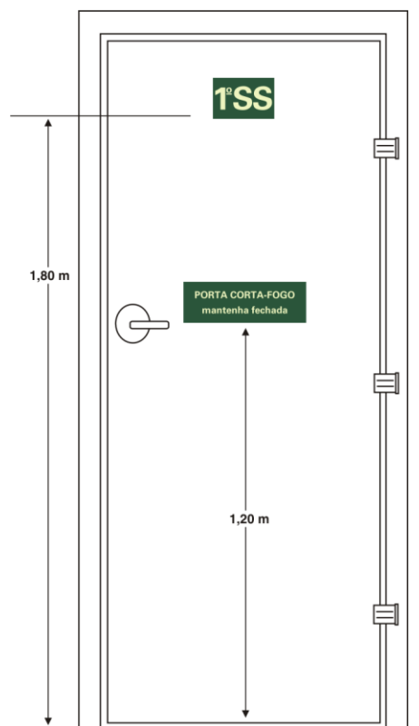
Figura 2 – Sinalização de porta Corta-fogo (vista do hall)
