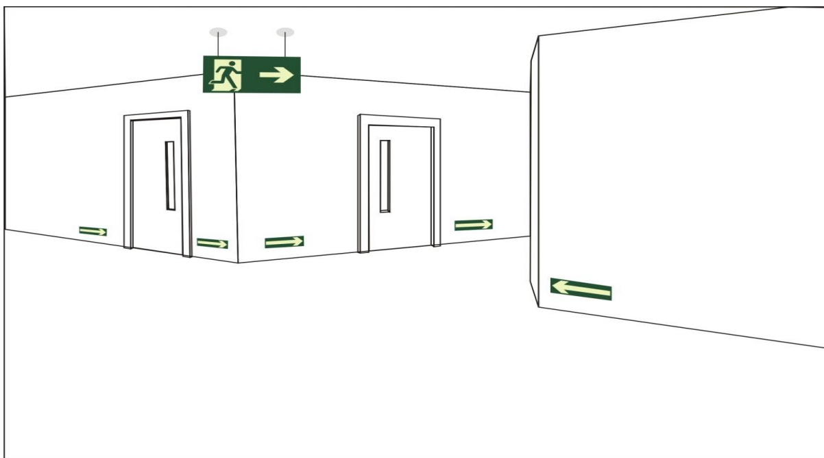
Figura 13 – Sinalização de saída perpendicular ao sentido da fuga, em dupla face.
