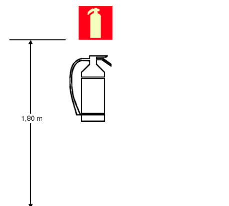
Figura 6 – Sinalização de extintores
