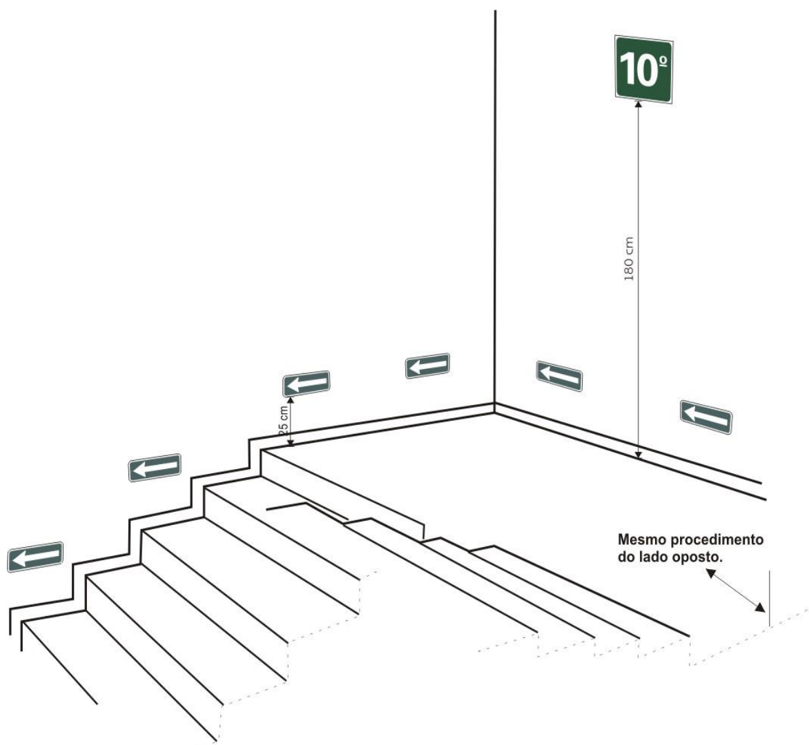
Figura 8 – Sinalização complementar. Exemplo de rodapé.
