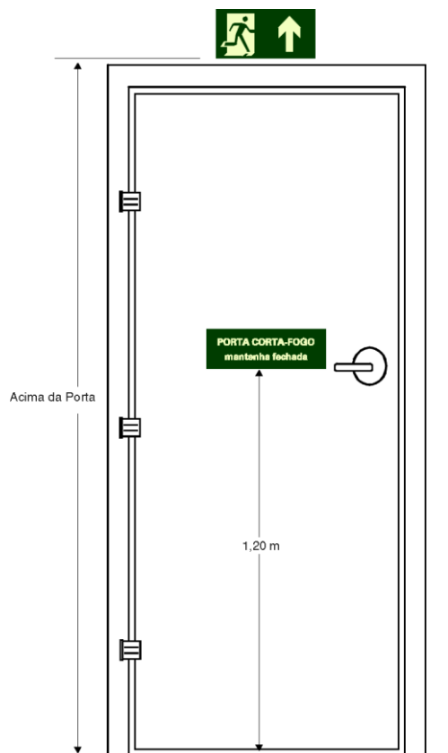
Figura 1 Sinalização de Porta Corta-fogo (vista da escada)
