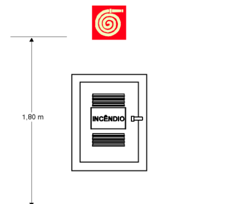
Figura 7 – Sinalização de hidrante
