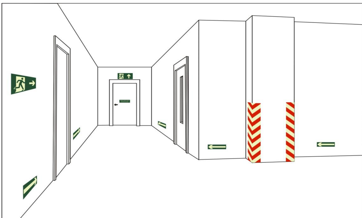
Figura 10 – Sinalização de saída sobre porta corta-fogo, sinalização complementar de saída e obstáculos.
