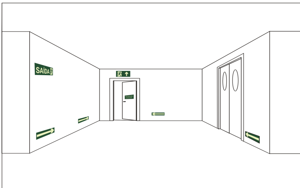
Figura 12 – Sinalização de saída sobre porta corta-fogo
