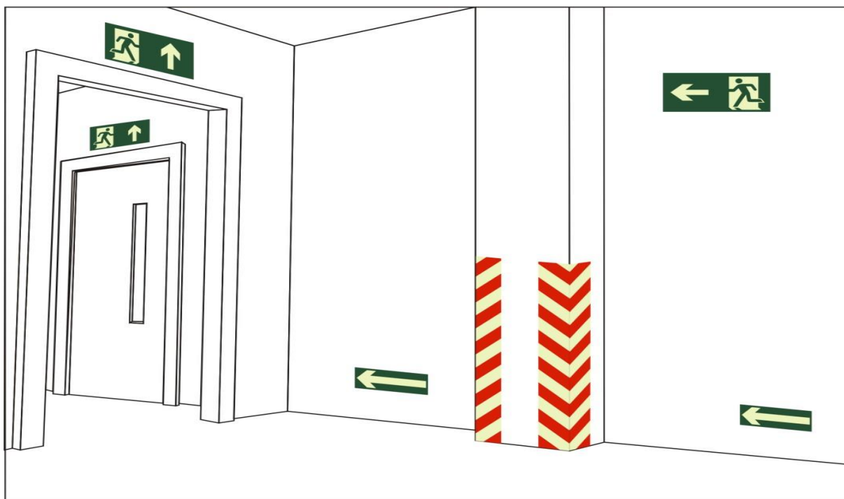
Figura 9 – Sinalização de saída sobre verga de portas, sinalização complementar de saídas e obstáculos.
