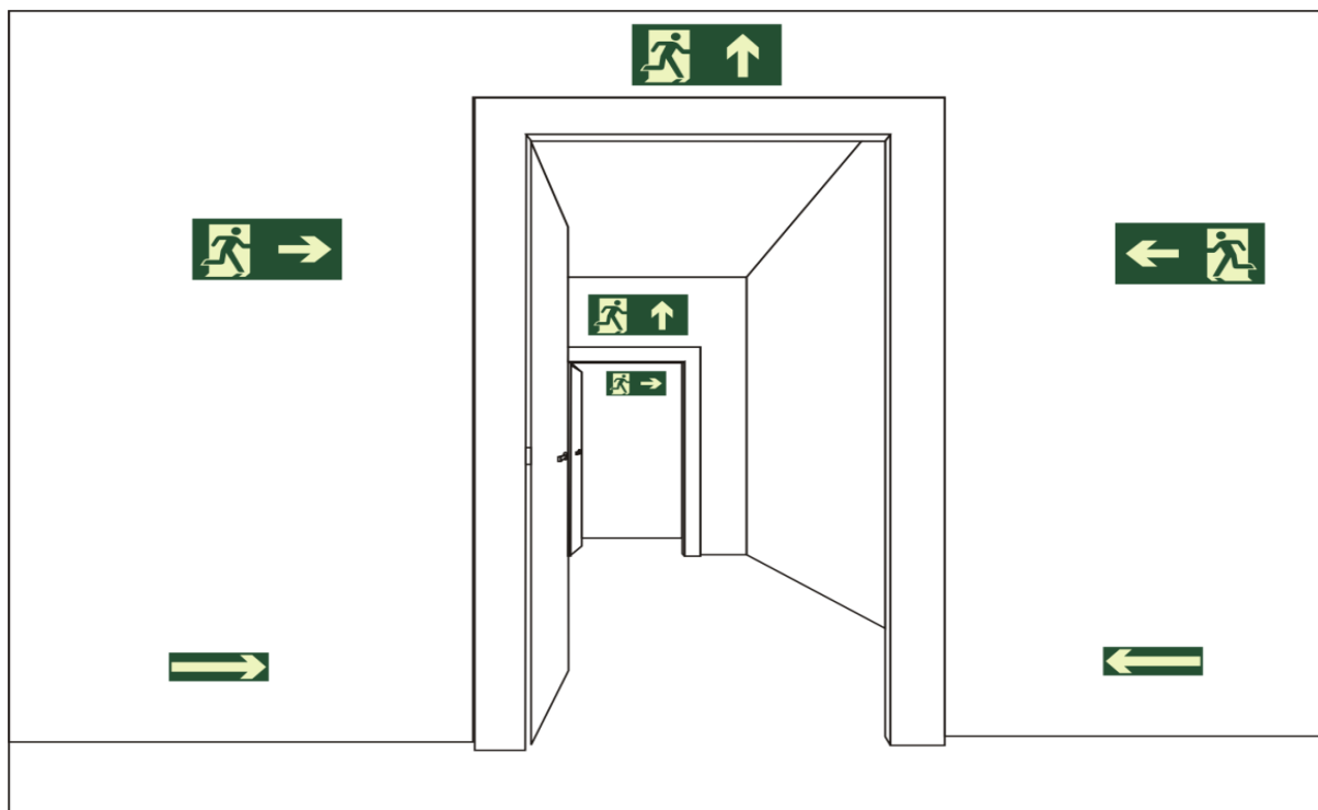
Figura 11 – Sinalização de saída sobre paredes e vergas de portas
