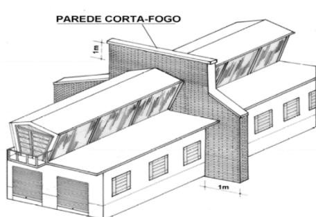
Figura 8 – Parede corta-fogo
