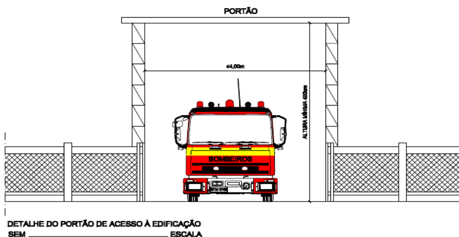
Figura 2 – Dimensões mínimas dos portões de acesso
